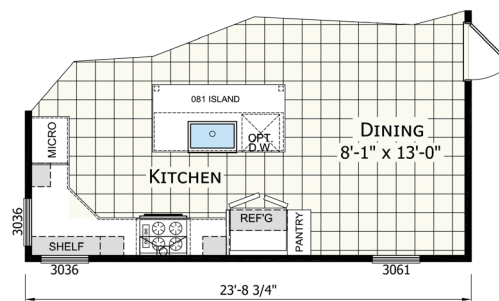
OPTIONAL UK2
